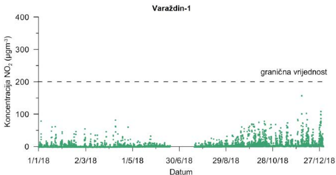
Slika 3: Vremenski niz satnih koncentracija NO 2 na mjernoj postaji Varaždin-1 tijekom 2018. godine
