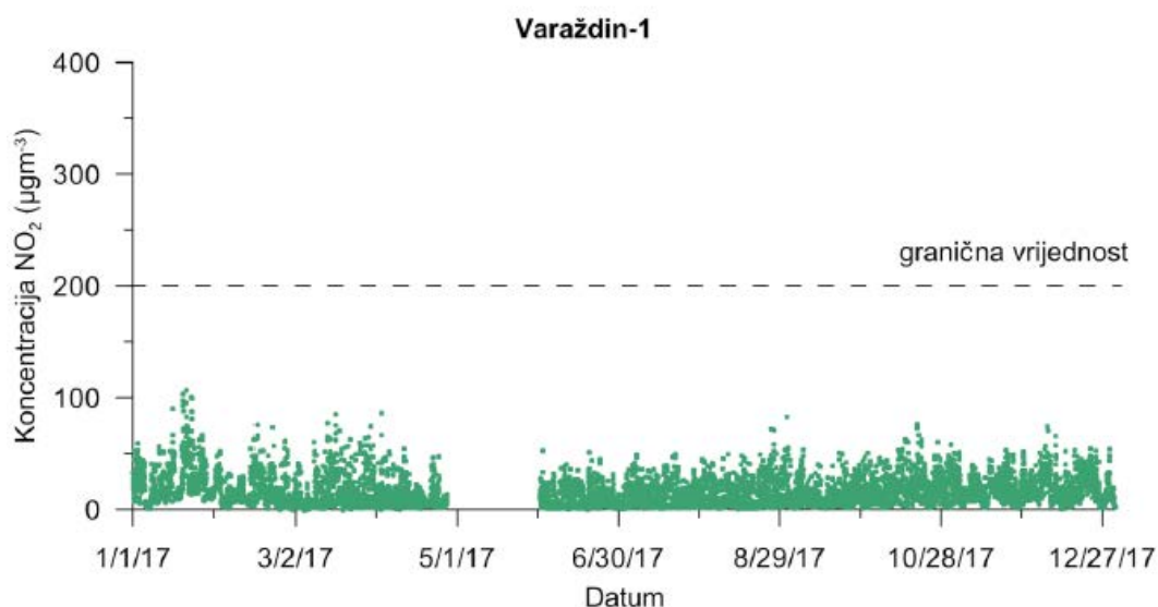
Slika 2: Vremenski niz satnih koncentracija NO 2 na mjernoj postaji Varaždin-1 tijekom 2017. godine
